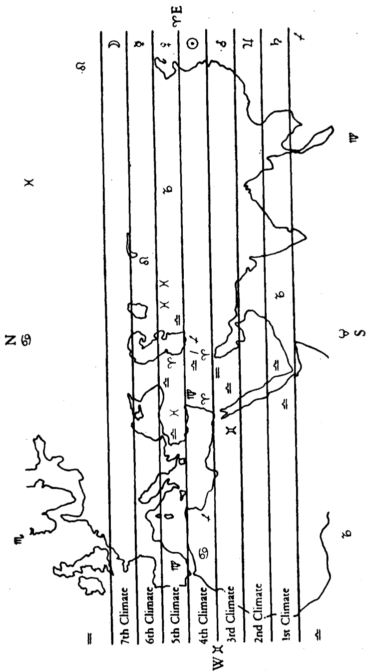
Рис.5. Астрологические управления, климаты и точки компаса по Аль-Бируни. (1029)
